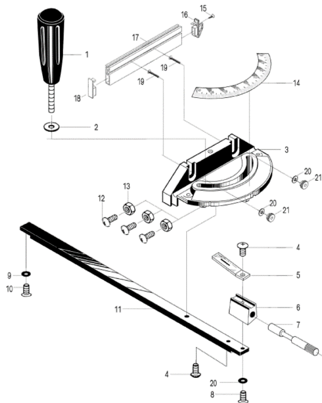
Рисунок 21. Упор угловой
