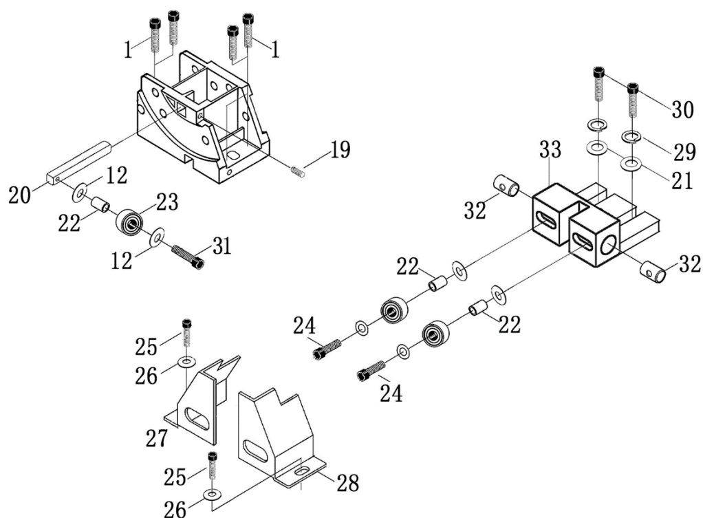
Рисунок 24. Блок нижних направляющих пыльного полотна
